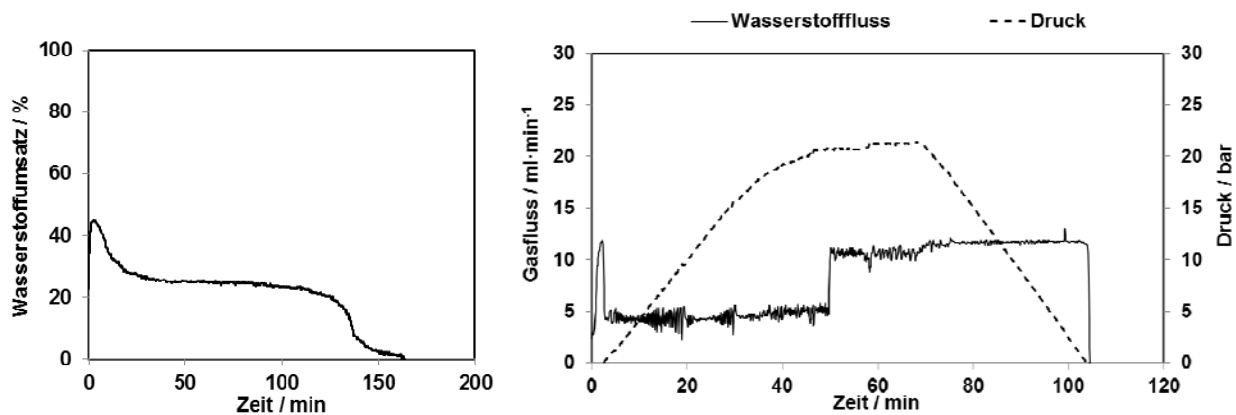
Abbildung 1: Links: repräsentative Reduktion von Magnetit zu Eisen. Die Reduktion wurde mit 25 \text{ ml} \cdot \text{min}^{-1} \text{ H}_2 bei 750^\circ \text{C} drucklos durchgeführt. Rechts: Gasfluss des freigesetzten Wasserstoffs und Systemdruck einer repräsentativen Dampf Oxidation bei 750^\circ \text{C} [4].
