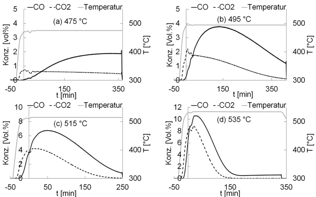
Abbildung 2: Verlauf der CO bzw. CO 2 -Konzentration bei 475 °C (a), 495 °C (b), 515 °C (c) und 535 °C (d). Es wurden jeweils 121 g Magnesit/Dolomit eingesetzt und bei einer Gaszusammensetzung von 90 Vol.% H 2 und 10 Vol.% N 2 (30 NL/h) am Reaktoreingang und Umgebungsdruck gearbeitet.
