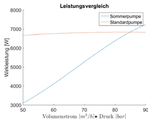
Abbildung 1: Pumpenvergleich
