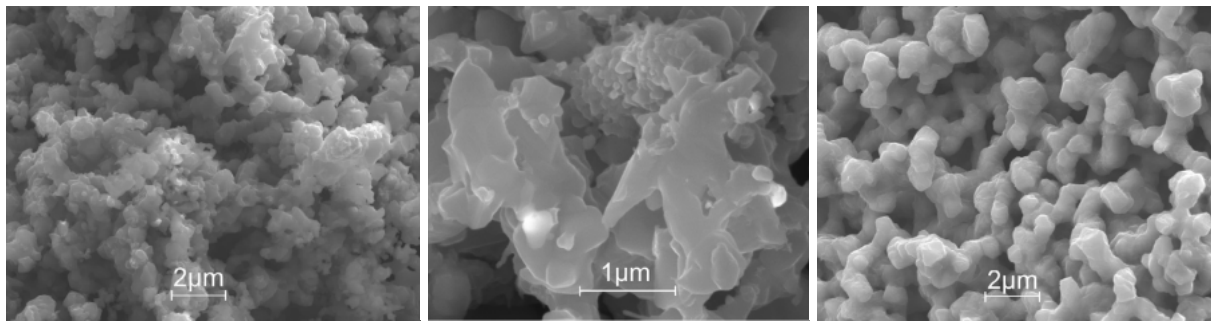
Abbildung 3: Rasterelektronenmikroskopische Aufnahmen der Kontaktmasse (90wt% \text{Fe}_2\text{O}_3 , 10wt% \text{Al}_2\text{O}_3 , 90-125 \mu\text{m} ) nach den Zyklenversuchen zur Freisetzung von Druckwasserstoff (links und Mitte). Rechts: Vergleichsprobe mit der gleichen Zusammensetzung nach 8 Zyklenversuchen unter atmosphärischem Druck und 750 °C [4].
