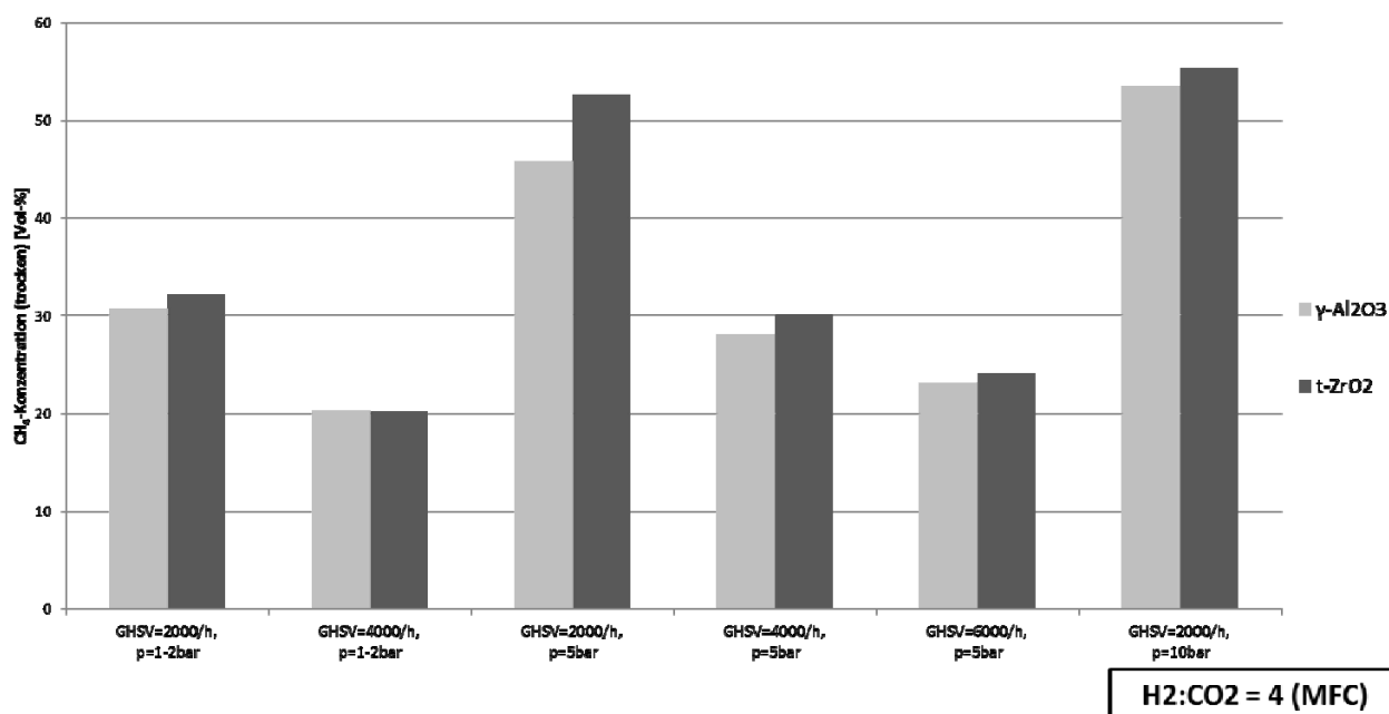
Abbildung 1: Erzielte \text{CH}_4 -Konzentration bei verschiedenen Versuchsbedingungen in Abhängigkeit des Trägermaterials; Gaszusammensetzung \text{H}_2:\text{CO}_2 = 4,0
