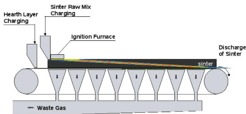
Abbildung 4: Wanderung der Heißtemperaturzone (= Brennfrent) durch das Sinterbett entlang der Fortbewegungsrichtung des Wanderrosts [6].
