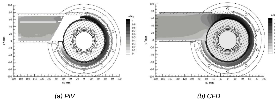
Abbildung 3: Normalisierte Geschwindigkeits-Konturdiagramme der Ebenen A und B
